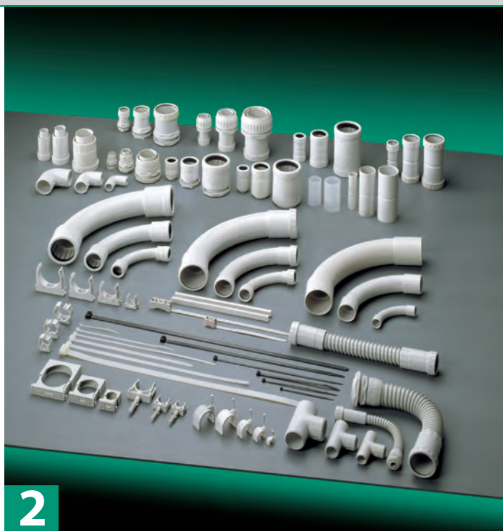
ACCESORIOS PARA TUBO Y FIJACIONES
